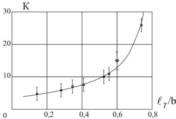
Рис. 14. Зависимость коэффициента К от протяженности трещины в пластине с неизменным током: l_T – длина трещины; b – ширина пластины. Радиус при вершине трещины a = \text{const} .
