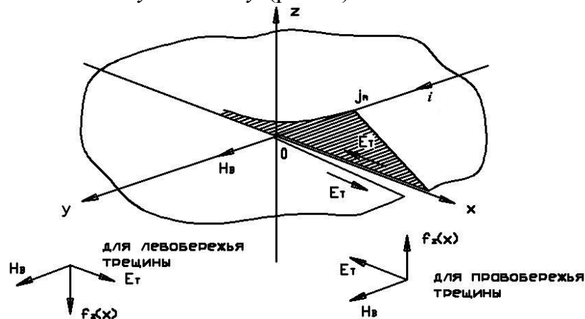
Рис. 9. Электромагнитная ситуация в пластине с трещиной. H_0 – напряженность внешнего магнитного поля; \ell_T – длина трещины; a – радиус при вершине, E_T – распределение напряженности электрического поля тока вдоль трещины.
