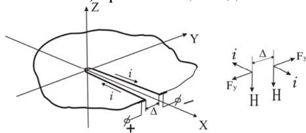
Рис. 1. Электромагнитная ситуация в пластине с трещиной при обтекании ее током i . \Delta - расстояние между берегами трещины, H - напряженность магнитного поля тока, F_y - пондеромоторная сила.
